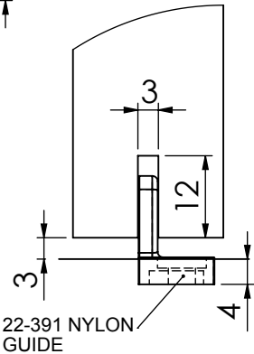
GUIDE SETUP FOR GROOVED DOOR
